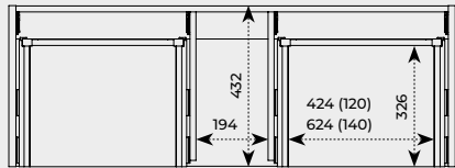
GÓRNA SZUFLADA KOMÓD
